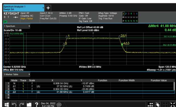
Figure 27 - 802.11ax HE40 SU Minimum 99% OBW
