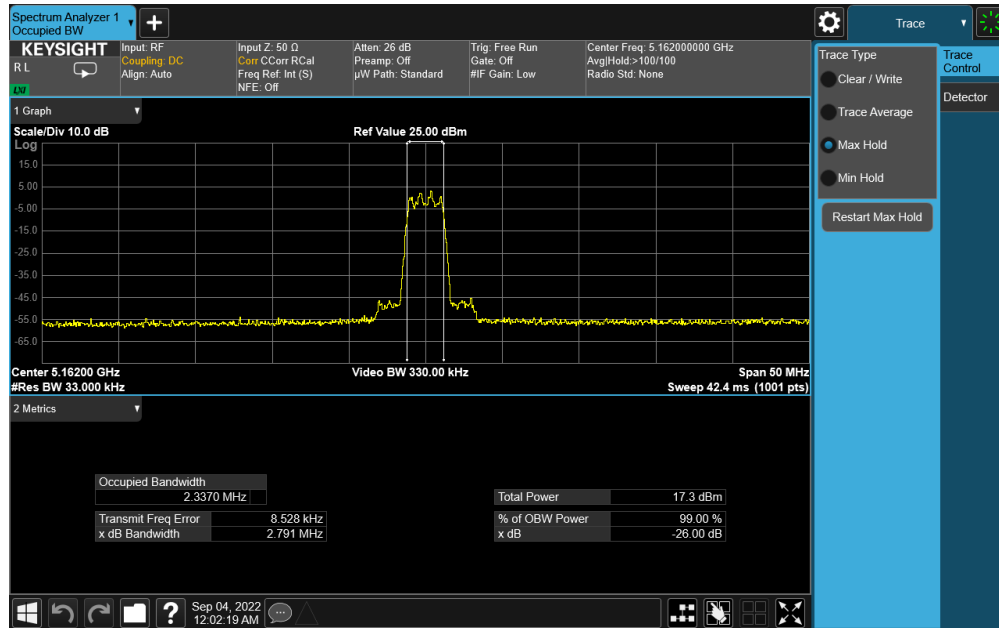
Plot 7-7. 26dB BW & 99% OBW Antenna 4a (HDR4, ePA, 5162MHz)
