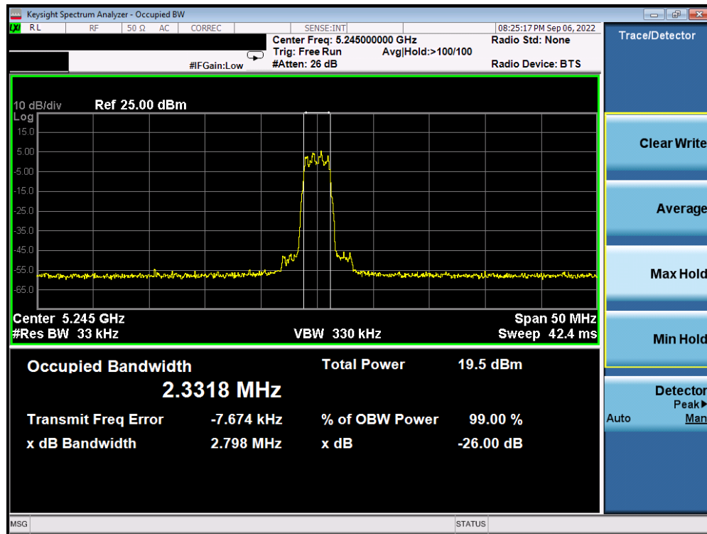
Plot 7-9. 26dB BW & 99% OBW Antenna WF5B (HDR4, ePA, 5245MHz)
