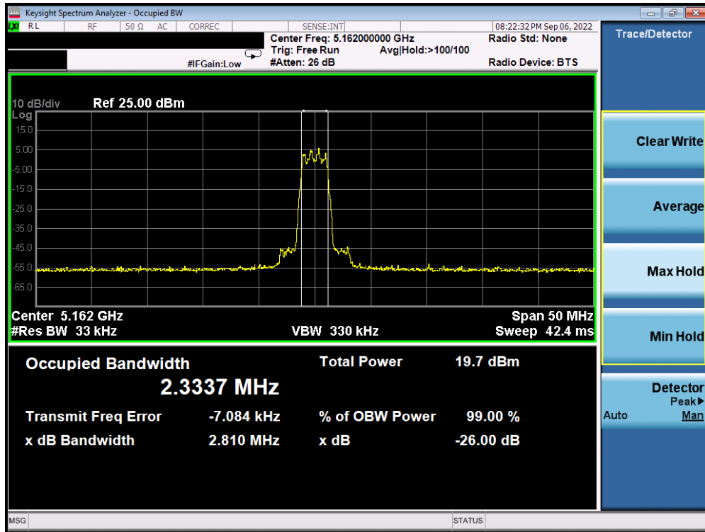
Plot 7-7. 26dB BW & 99% OBW Antenna WF5B (HDR4, ePA, 5162MHz)
