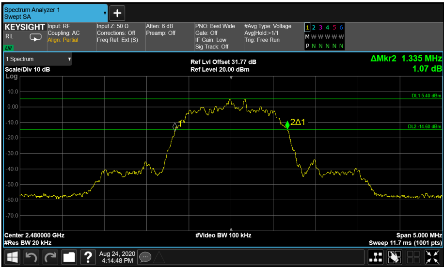
Figure 17 - Core 2 \pi/4 DQPSK 2480 MHz (CH78)
