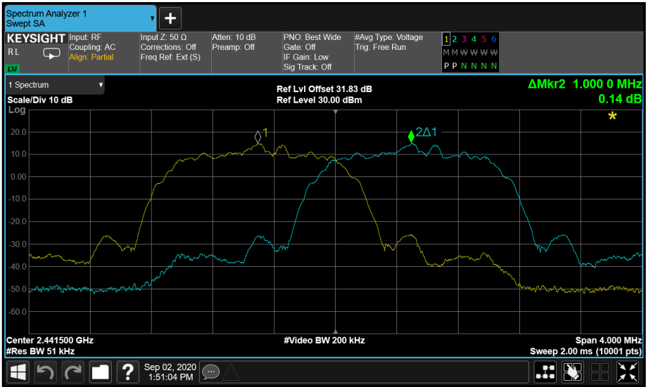
Figure 3 - \pi/4 DQPSK - 2441 MHz (CH 39)
