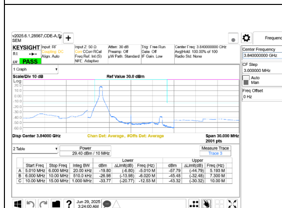
5G NR n77 10MHz BPSK Mid Channel RB1-0 Port A+B
