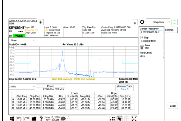
5G NR n41 20MHz BPSK Middle Channel RB1-0 Port A+B
