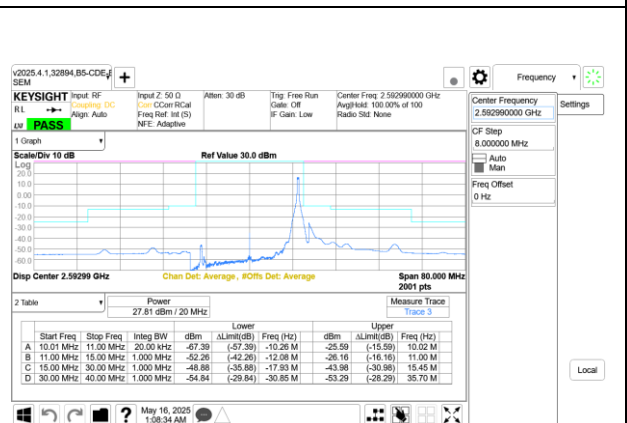
5G NR n41 20MHz BPSK Mid Channel RB1-50 Port A+B
