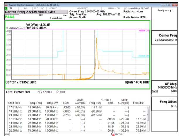
5G NR n41 35MHz BPSK Low Channel RB1-91
