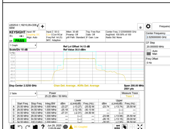
5G NR n7 50MHz BPSK Low Channel RB270-0
