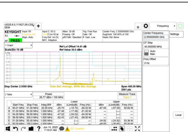
5G NR n41 100MHz BPSK Low Channel RB1-0
