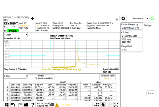
5G NR n41 60MHz BPSK Low Channel RB1-161
