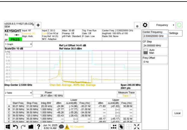
5G NR n41 60MHz BPSK Low Channel RB1-0
