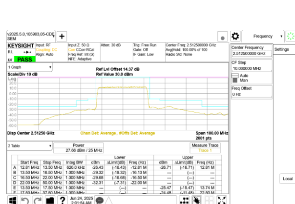
5G NR n41 25MHz BPSK Low Channel RB64-0
