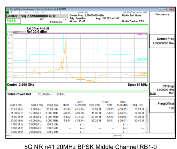
5G NR n41 20MHz BPSK Middle Channel RB1-0
