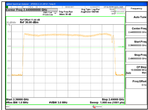
100MHz SPAN
