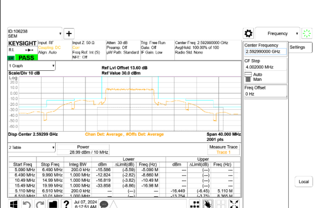
5G NR n41 10MHz BPSK Middle Channel RB24-0
