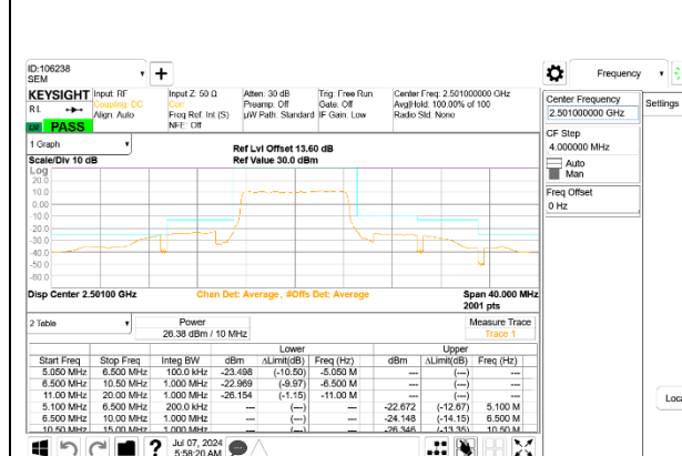
5G NR n41 10MHz BPSK Low Channel RB24-0
