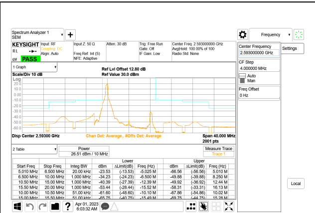
5G NR n41 10MHz BPSK Middle Channel RB1-0, ID:19210
