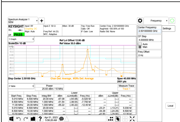
5G NR n41 10MHz BPSK Low Channel RB1-23, ID:19210
