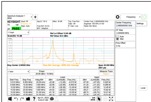
5G NR n41 10MHz BPSK High Channel RB1-0, ID:19210
