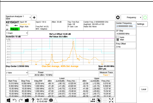
5G NR n41 10MHz BPSK Middle Channel RB1-23, ID:19210
