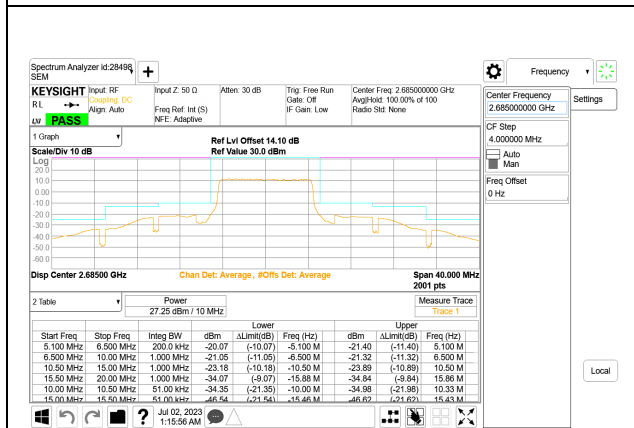
5G NR n41 10MHz BPSK High Channel RB24-0
