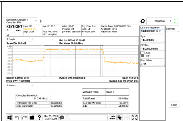
5G NR n77 70MHz BPSK Middle Channel RB180-0 ID:28498
