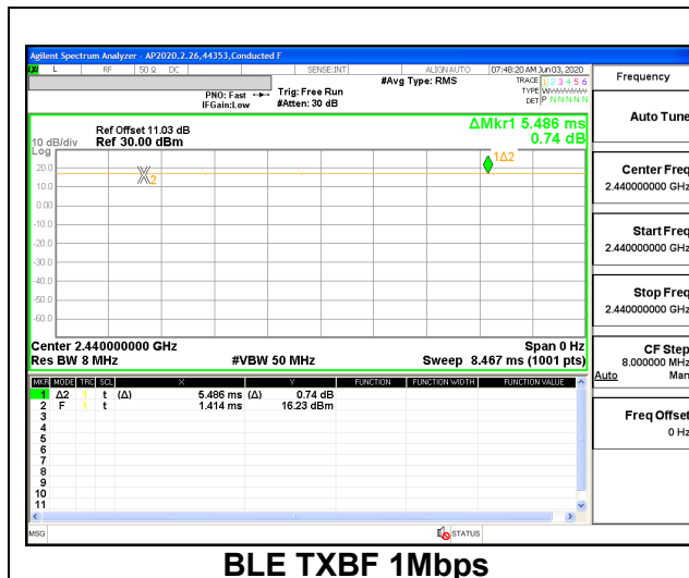
BLE 1Mbps
