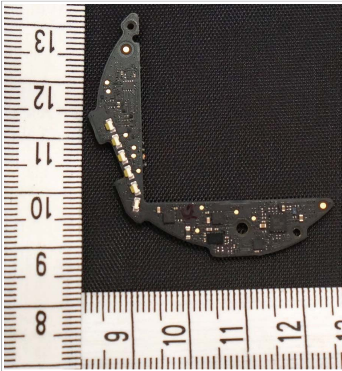
Right PCB
