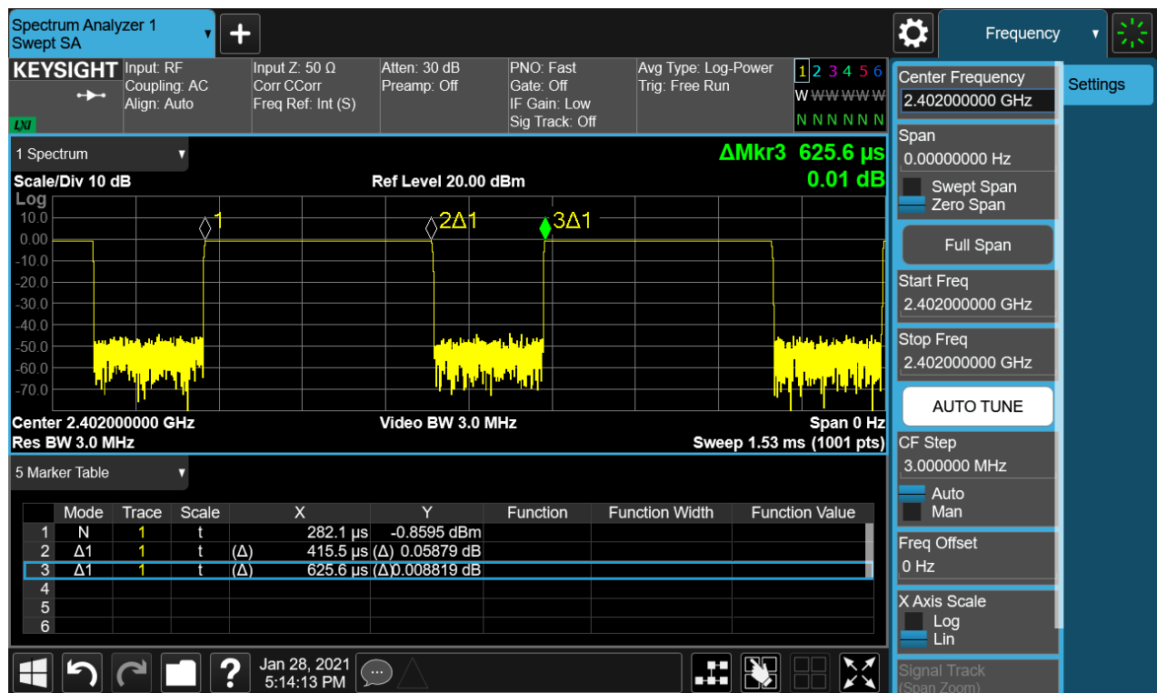
BLE 1Mbps
