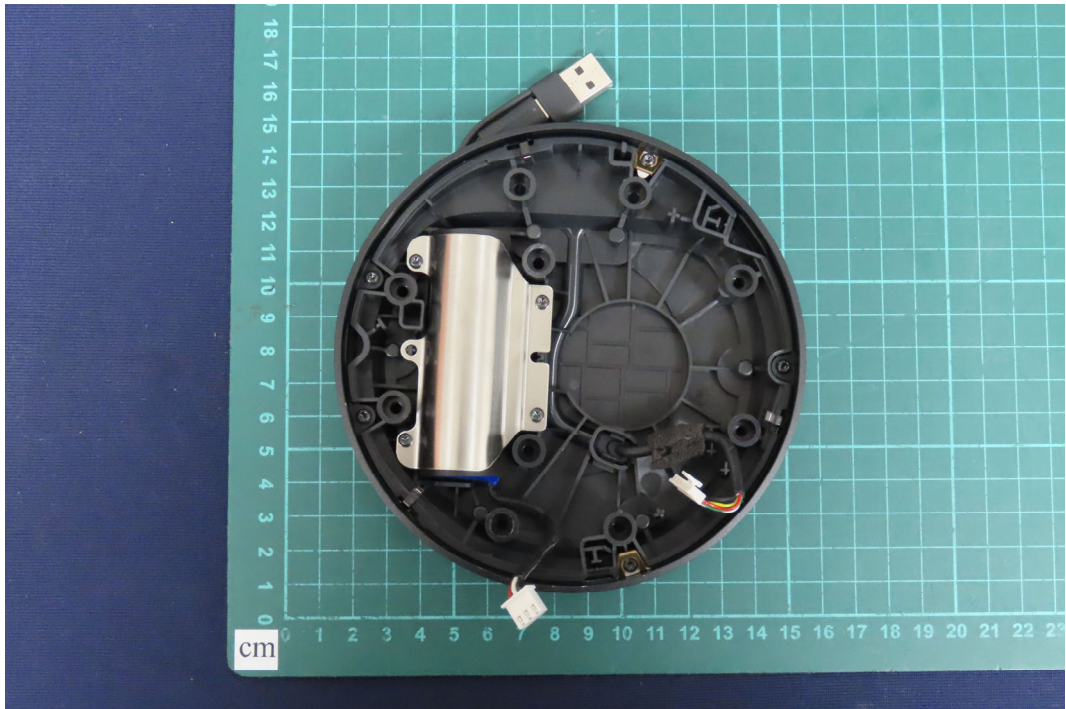
(20) EUT Photo
