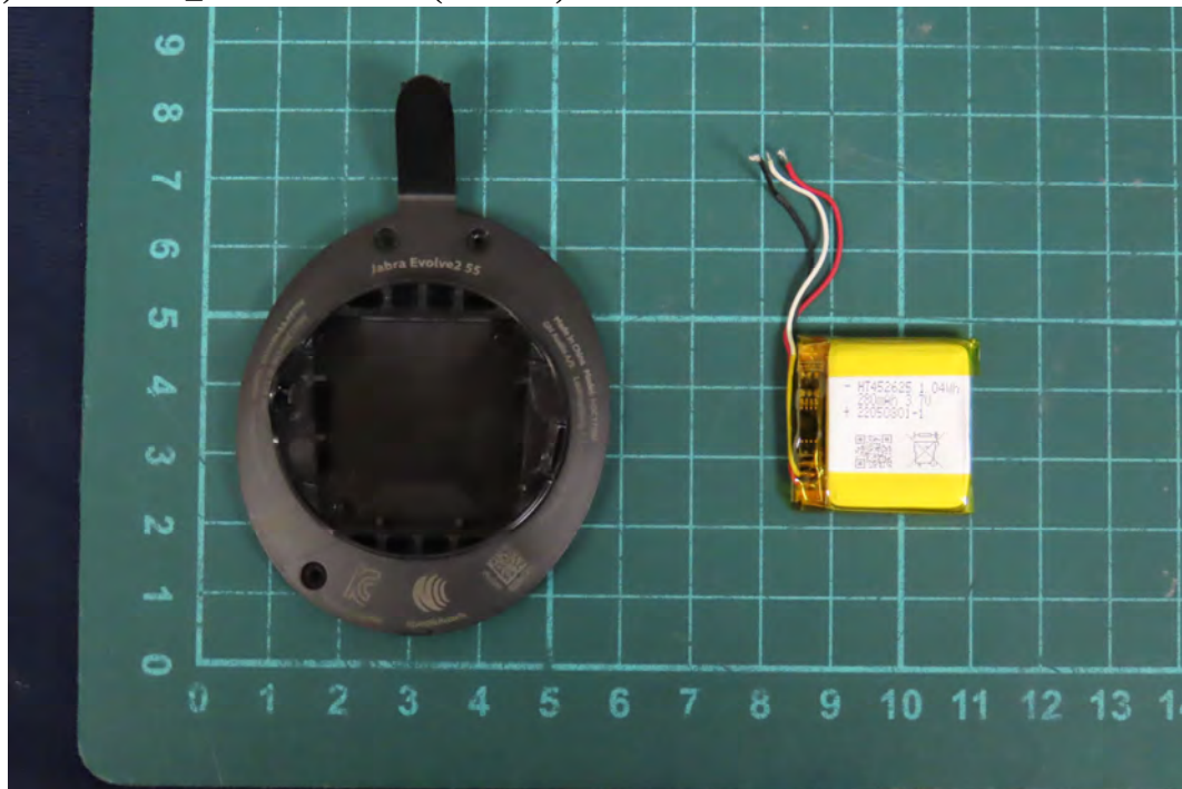
(13) EUT Photo _M/N: HSC170W (Binaural)
