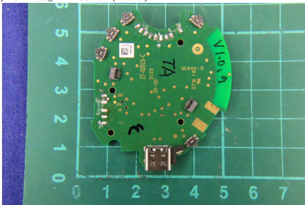
(20) EUT Photo _M/N: HSC170W (Binaural)
