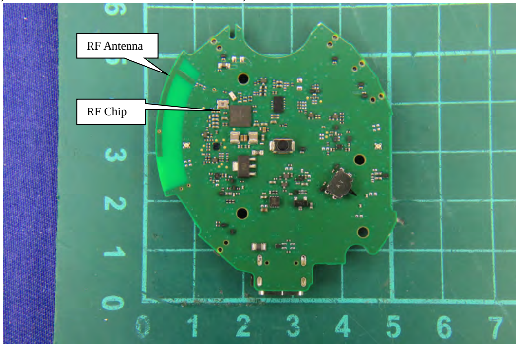
(21) EUT Photo _M/N: HSC170W (Binaural)
