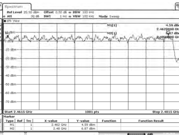
2462-2480MHz
