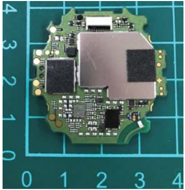
Module Front side
