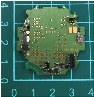
Module Back side
