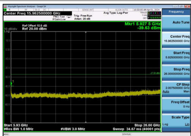
U-NII-3 ,Plot 3,5925MHz~26000MHz-802. 11ac(80MHz),5775MHz,Ant1
