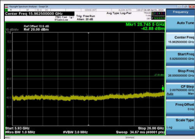
U-NII-3 ,Plot 3,5925MHz~26000MHz-802. 11ac(40MHz),5795MHz,Ant1
