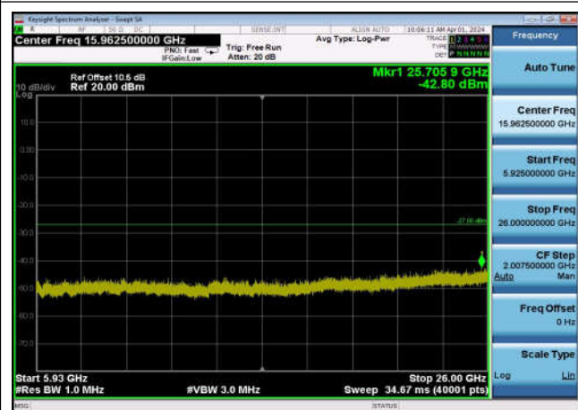
U-NII-3 ,Plot 3,5925MHz~26000MHz-802. 11ac(20MHz),5825MHz,Ant1
