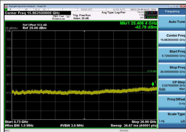
U-NII-2c ,Plot 3,5725MHz~26000MHz-802 .11ac(40MHz),5670MHz,Ant1
