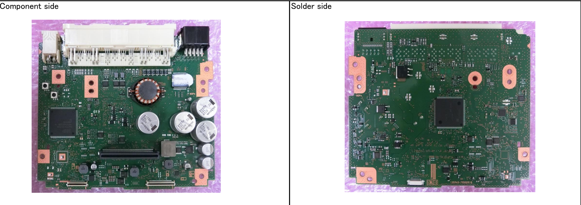
【AUDIO Board】
