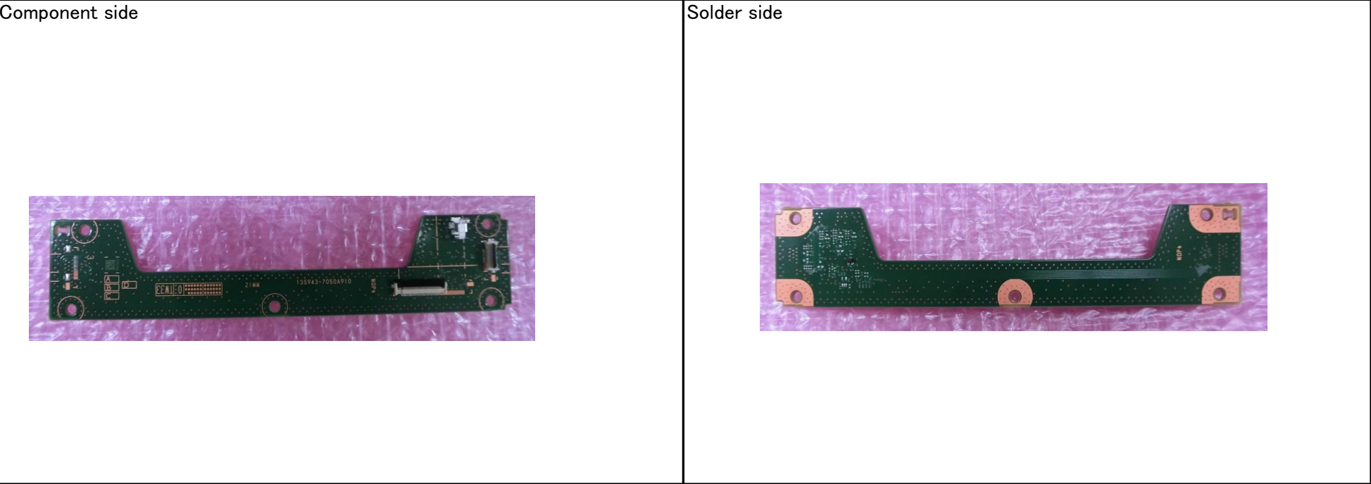
【SW Board】
