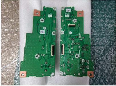
【V-IF Board】
