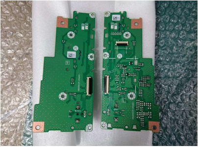
【V-IF Board】
