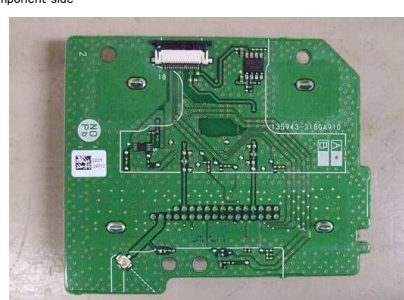
【XM Board】
