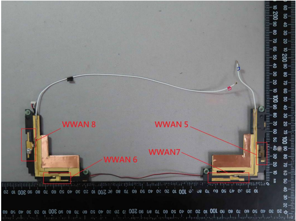
WWAN Antenna
