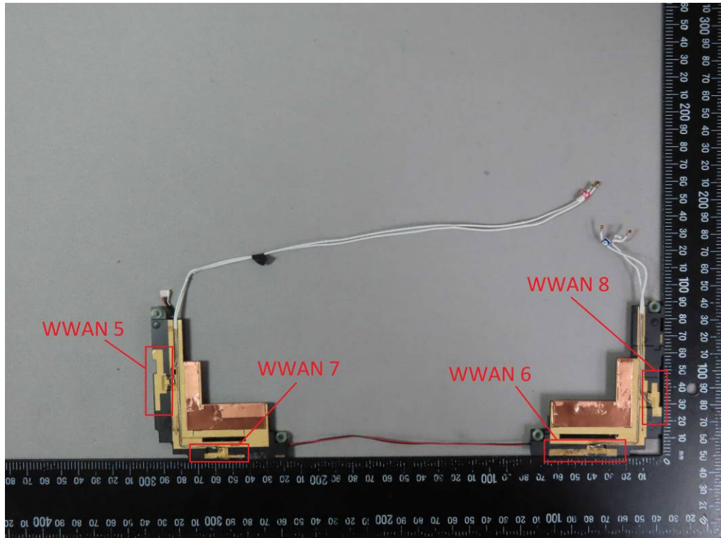
WWAN Antenna
