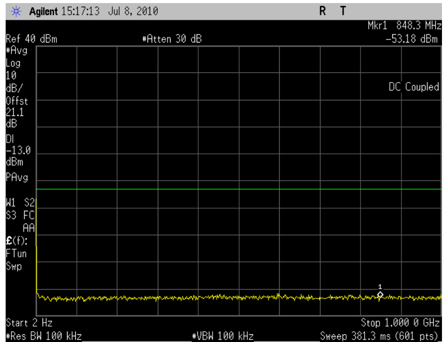
Plot 7.2 -12 (GMSK Ch810)
