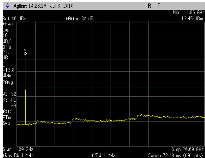
Plot 7.2 -8 (GMSK Ch512)
