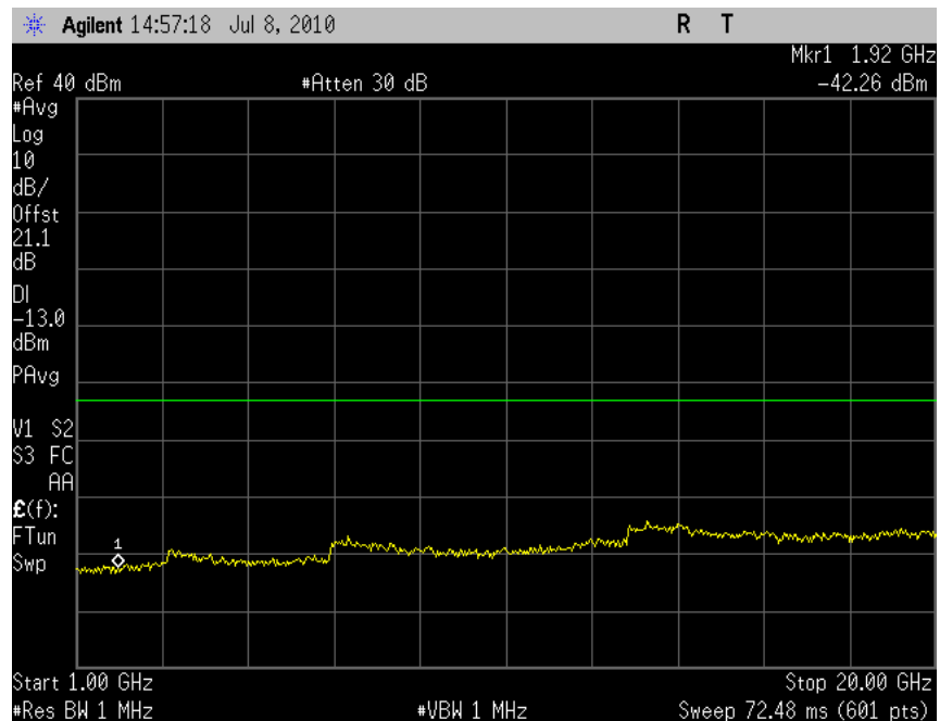
Plot 7.2 - 2 (GMSK Ch128)
