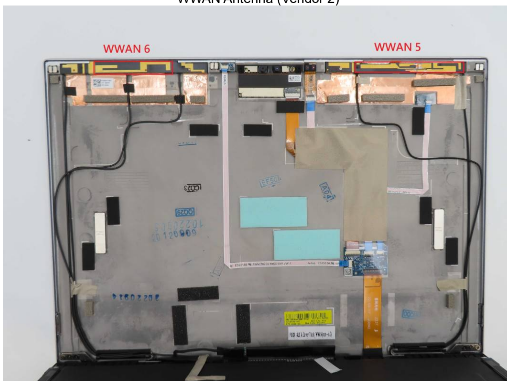
WWAN Antenna (Vendor 2)
