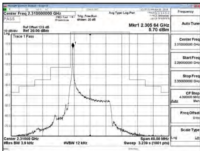
Band30_10MHz_QPSK_1_49_CH27710
