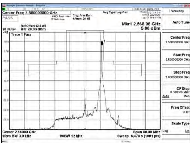
Band7_20MHz_16QAM_1_99_CH21350
