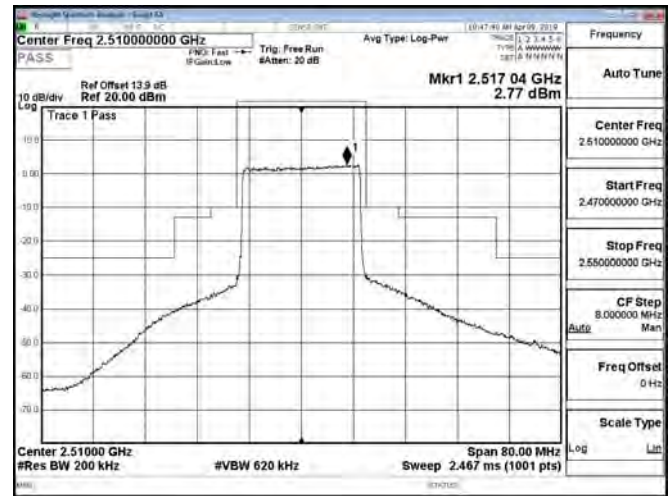
Band7_20MHz_16QAM_100_0_CH21100
