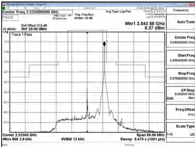
Band7_20MHz_16QAM_1_99_CH21350
