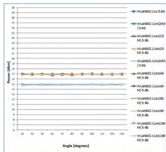
5.6GHz Tx2(SISO)
