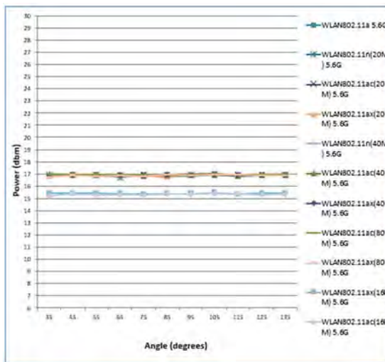
5.6GHz Tx1(SISO)
