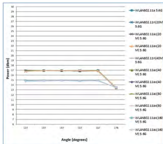
5.6GHz Tx2(SISO)
