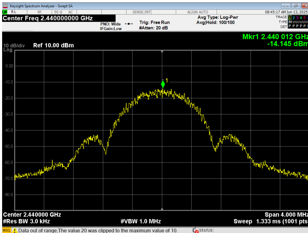
15 PSD, BLE 1MB, 2440MHz
