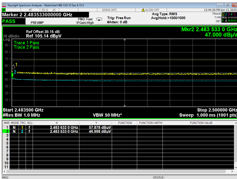
20 HBE Restricted, BLE 2MB, 2480MHz
