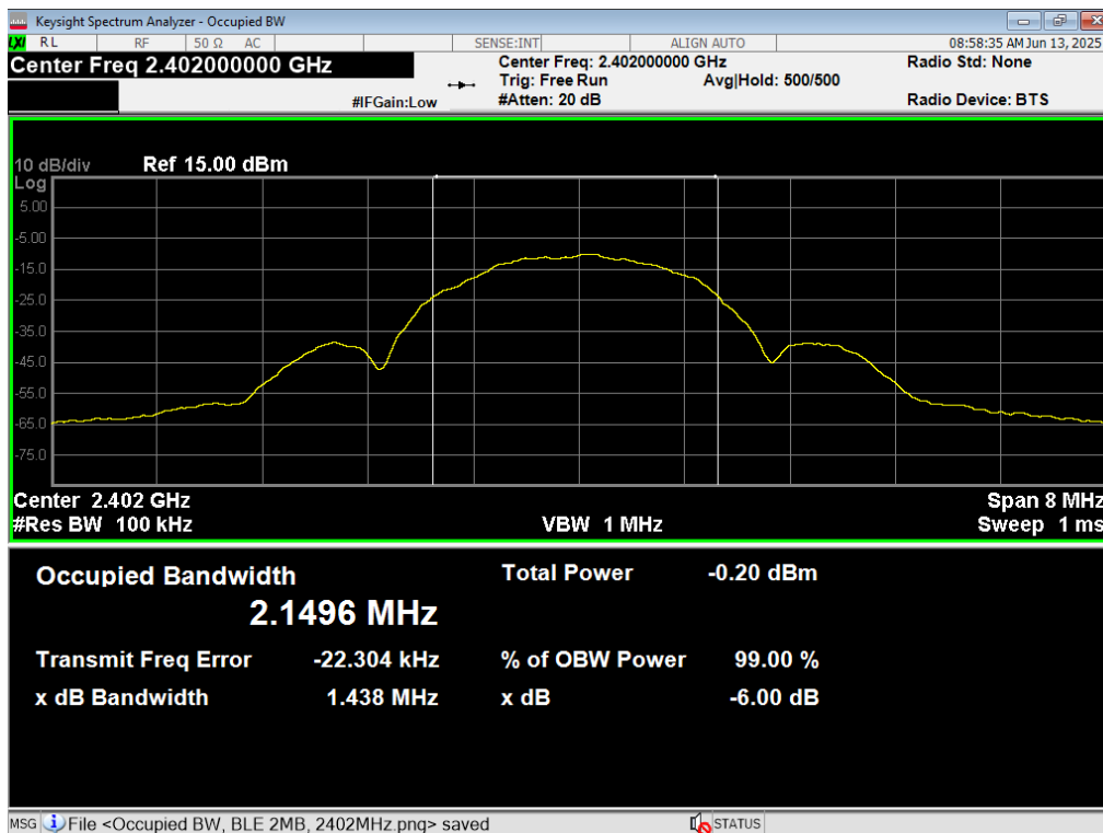
17 6dB BW, BLE 2MB, 2402MHz
