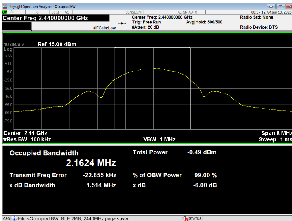
18 6dB BW, BLE 2MB, 2440MHz
