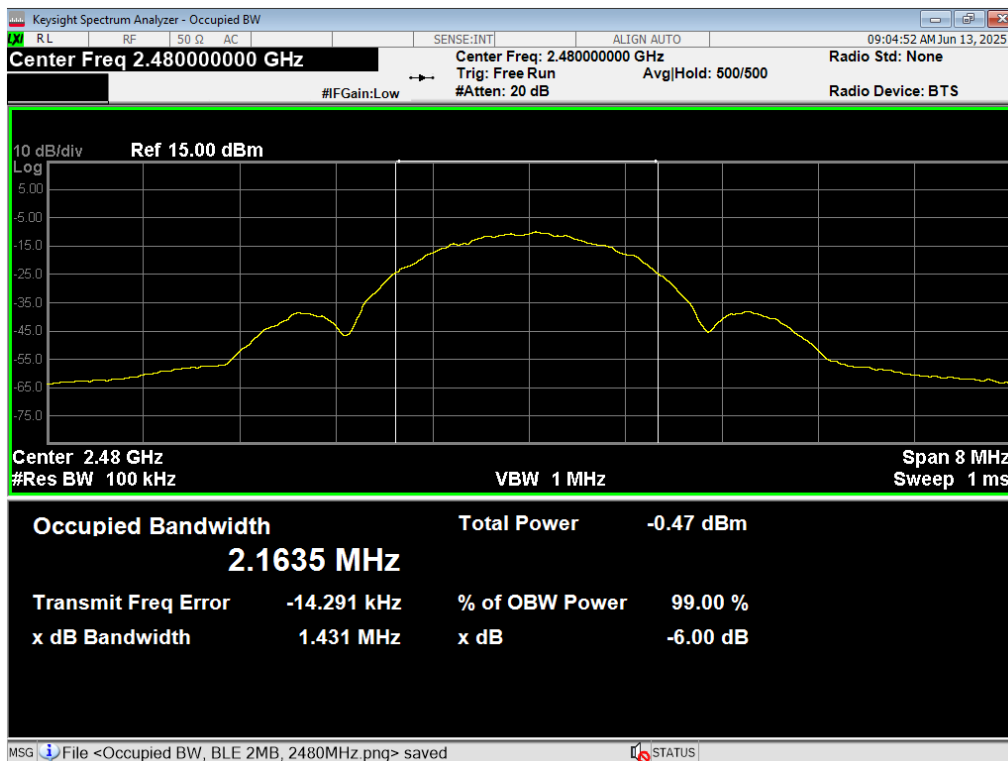
19 6dB BW, BLE 2MB, 2480MHz
