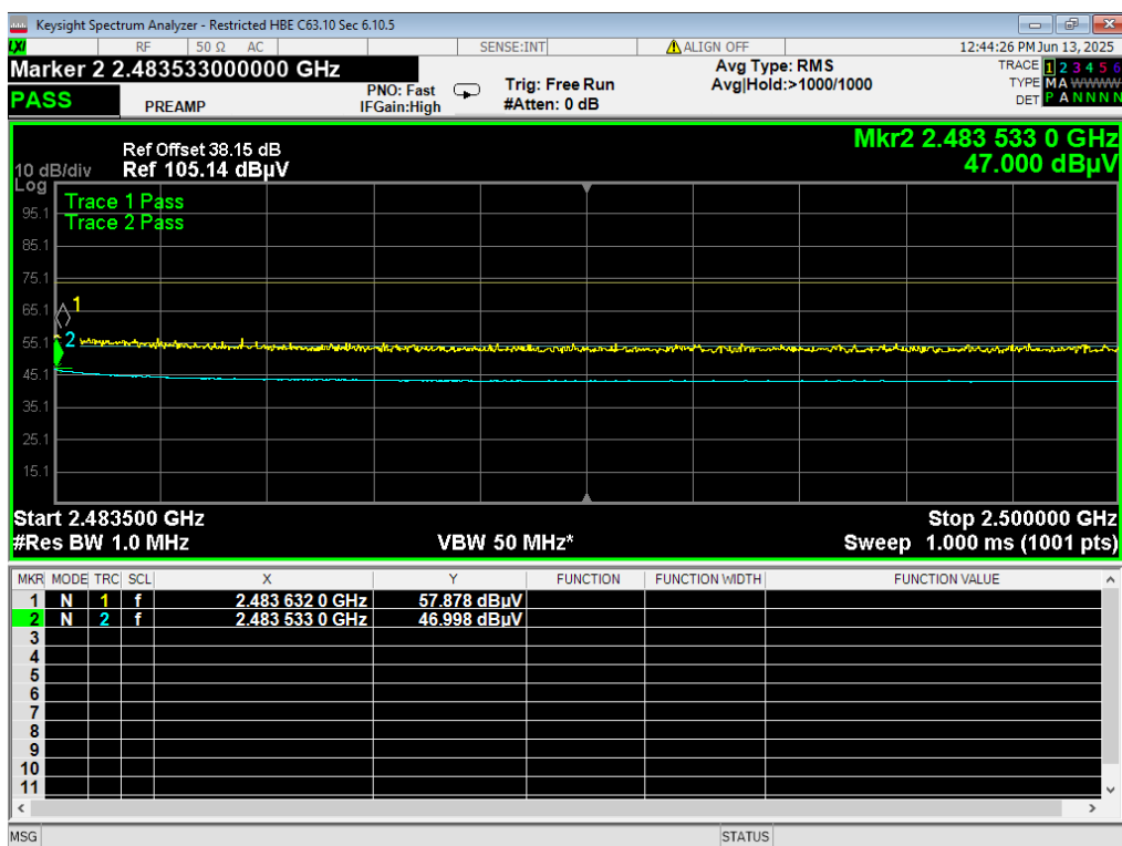
20 HBE Restricted, BLE 2MB, 2480MHz
