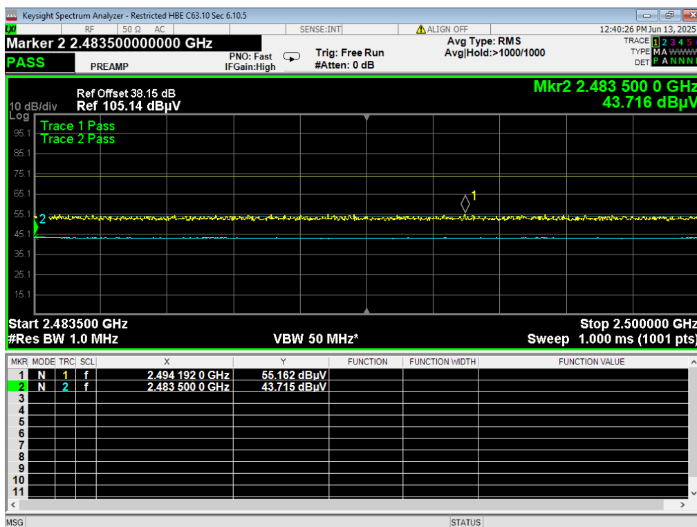
04 HBE Restricted, BLE 1MB, 2480MHz
