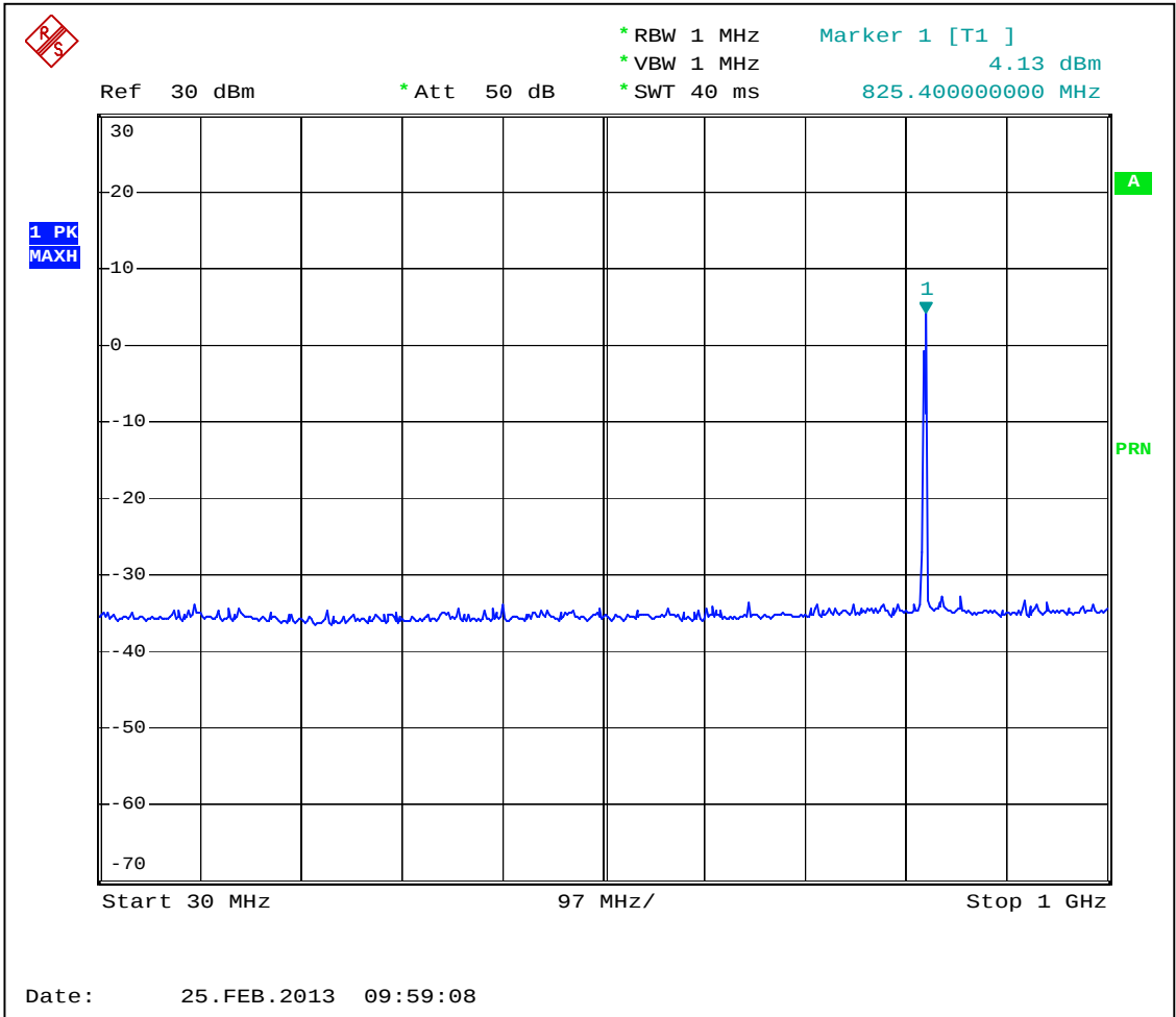
Graph 3.5.1
