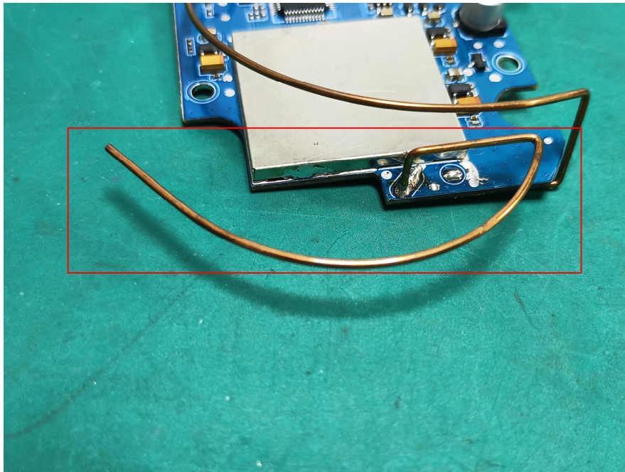
2.4GHz Antenna
