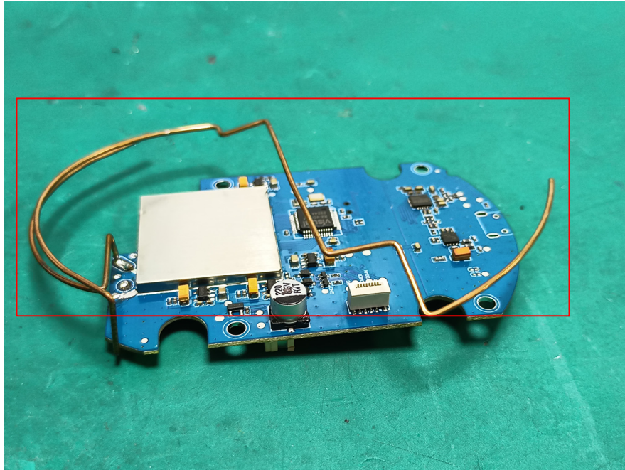
900MHz Antenna
