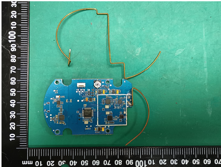
2.4GHz Antenna
