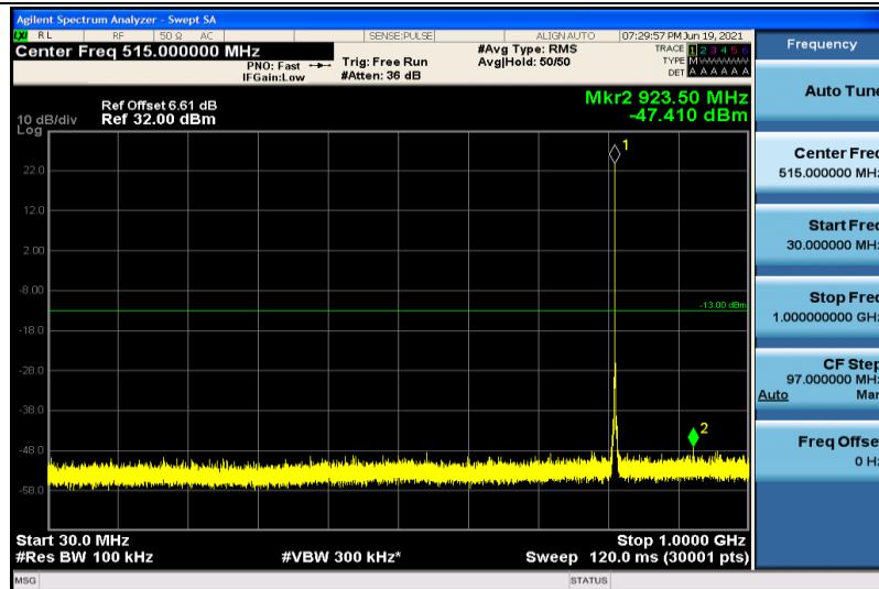
Band26-1.4MHz-QPSK-26697-1RB#0-30~1000MHz
