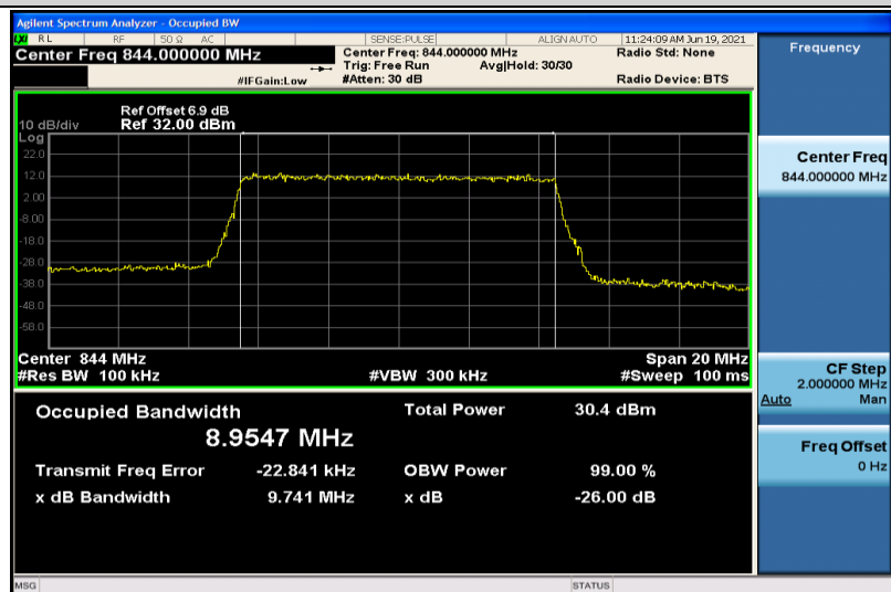
Band5-10MHz-QPSK-20600-50RB#0-8.9547
