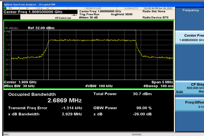
Band2-3MHz-QPSK-19185-15RB#0-2.6869
