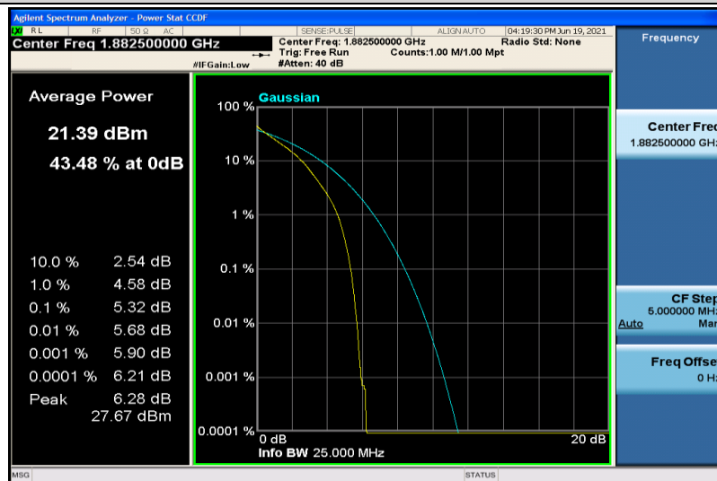
Band25-5MHz-QPSK-26365-25RB#0
