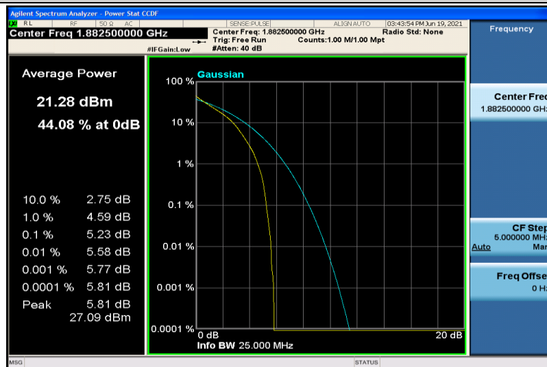
Band25-1.4MHz-QPSK-26365-6RB#0
