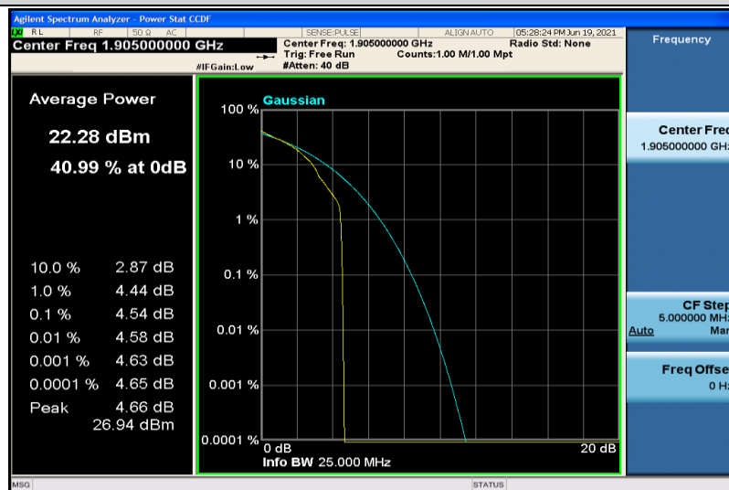
Band25-20MHz-QPSK-26590-1RB#0
