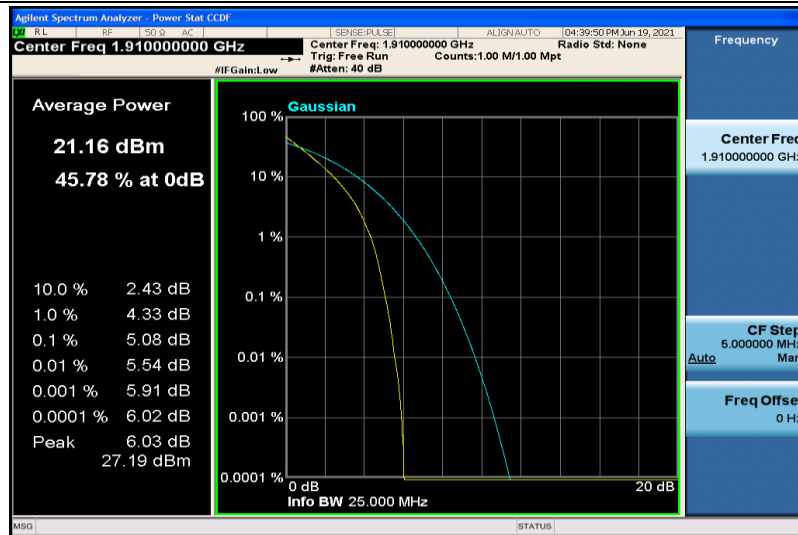
Band25-10MHz-QPSK-26640-50RB#0
