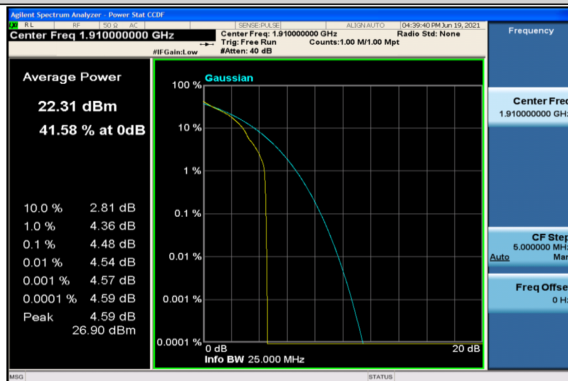
Band25-10MHz-QPSK-26640-1RB#0
