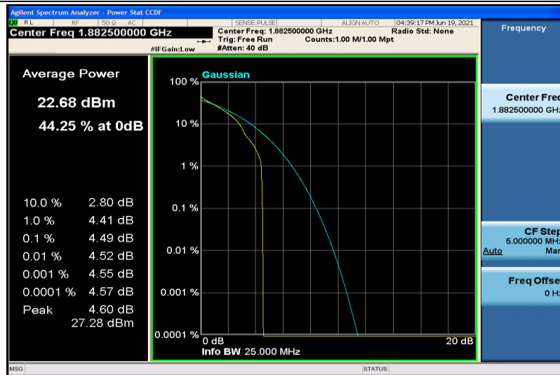
Band25-10MHz-QPSK-26365-1RB#0
