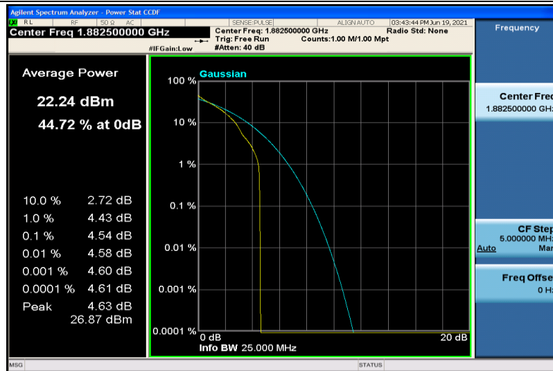
Band25-1.4MHz-QPSK-26365-1RB#0
