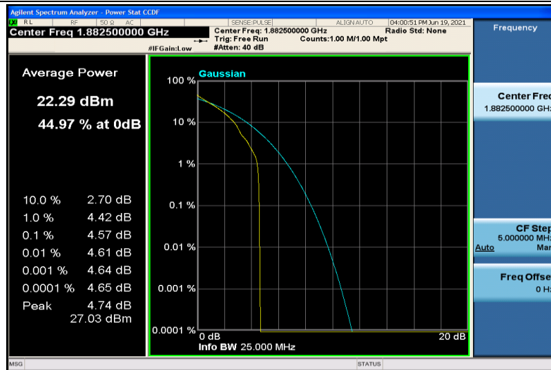
Band25-3MHz-QPSK-26365-1RB#0
