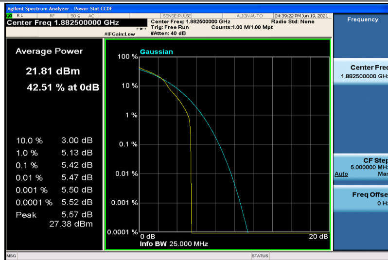
Band25-10MHz-16QAM-26365-1RB#0
