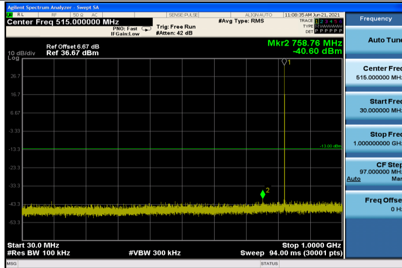
GPRS850-128-30~1000
