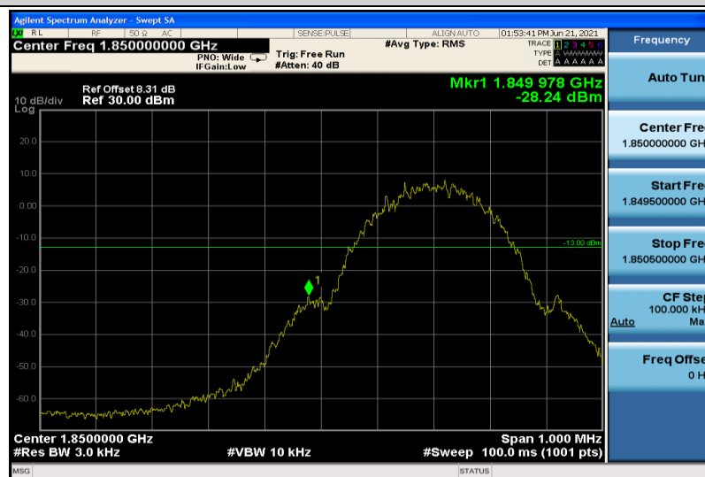
GPRS1900-512
