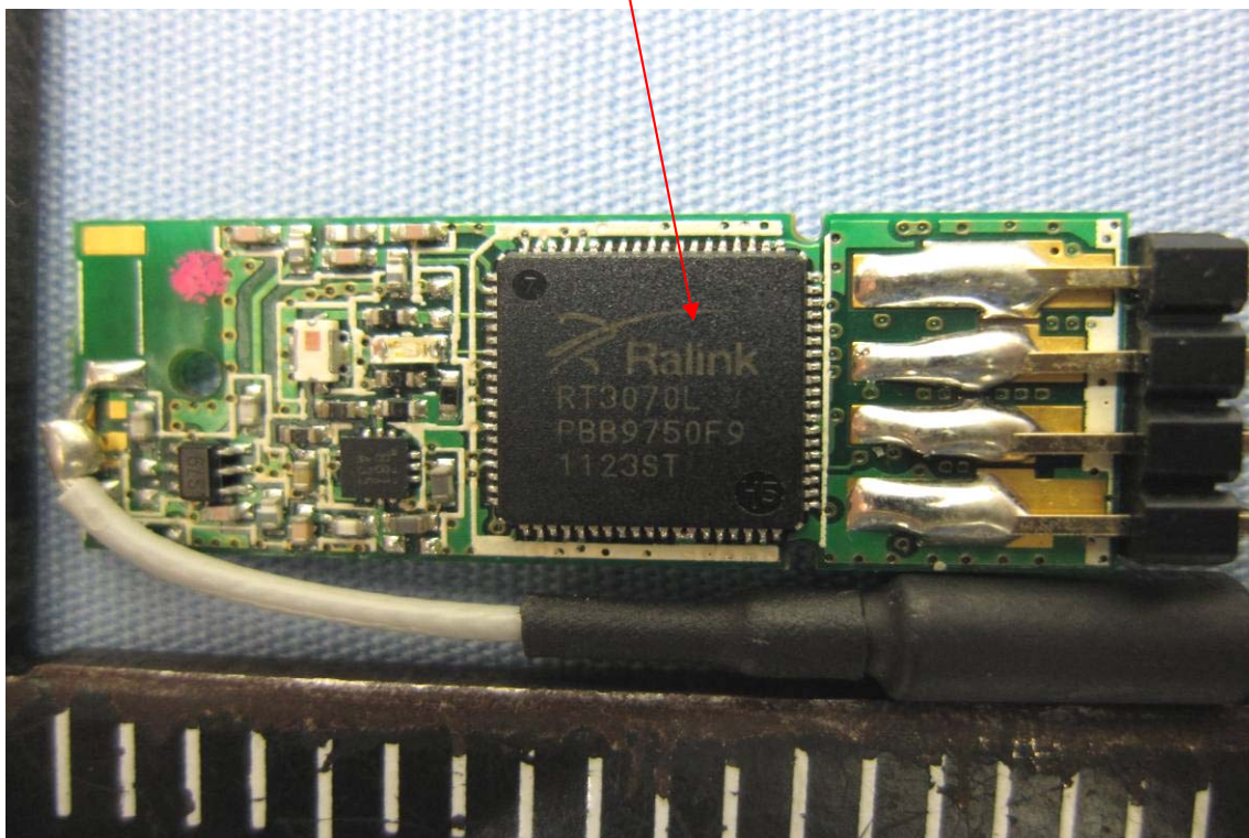
WLAN Module
