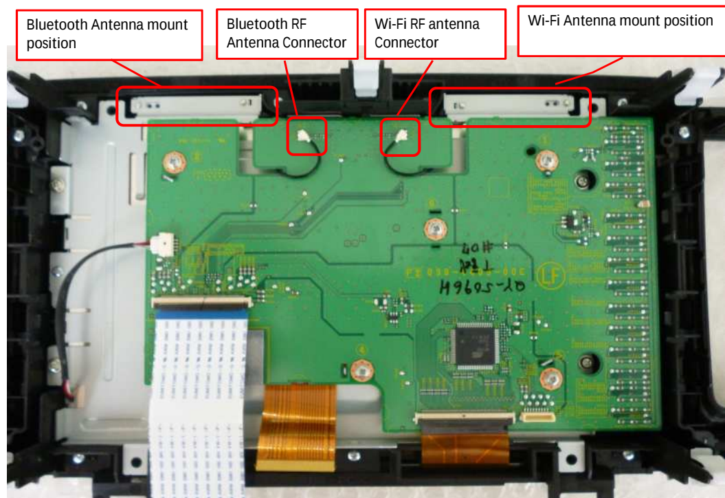
LCD PCB ASSY - F1 View
