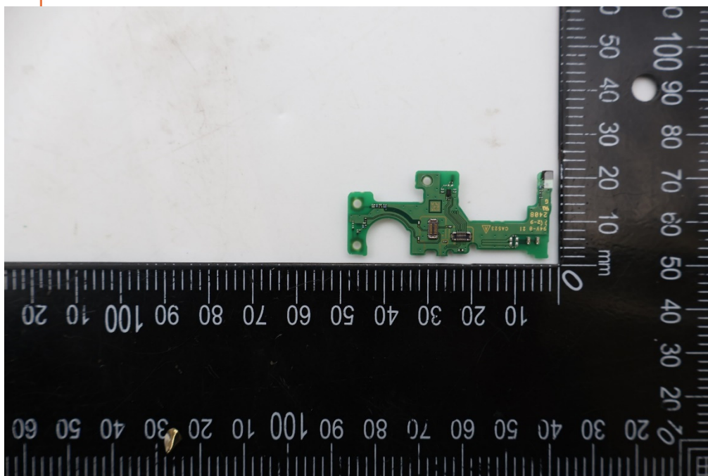
NFC Antenna
