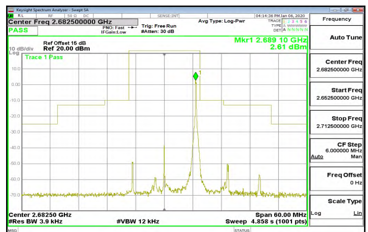
Band41_15MHz_QPSK_1_74_CH41515
