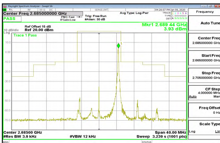
Band41_10MHz_QPSK_1_49_CH41540
