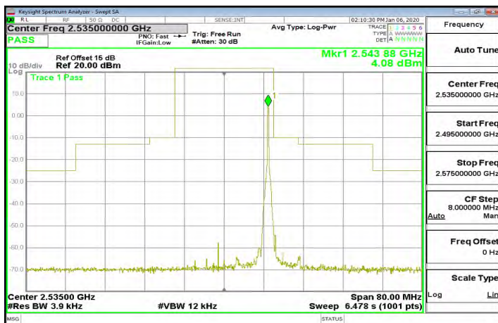
Band7_20MHz_64QAM_1_99_CH21350
