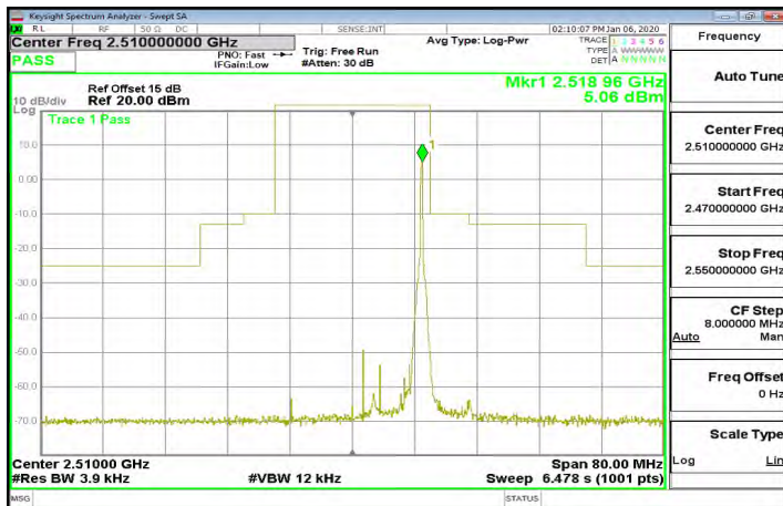
Band7_20MHz_64QAM_1_99_CH21100
