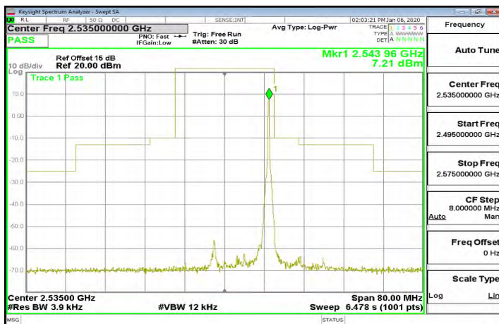
Band7_20MHz_QPSK_1_99_CH21350
