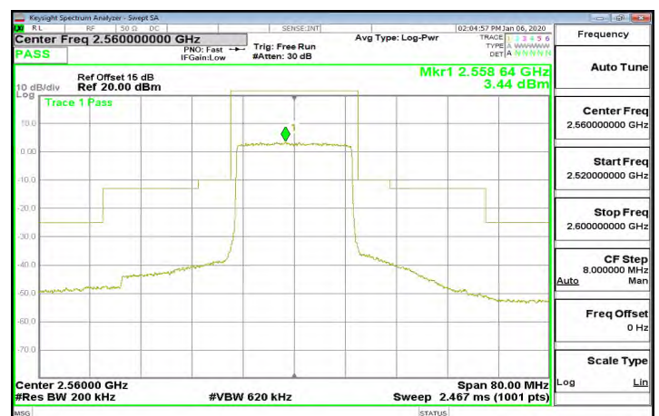
Band7_20MHz_QPSK_100_0_CH21350
