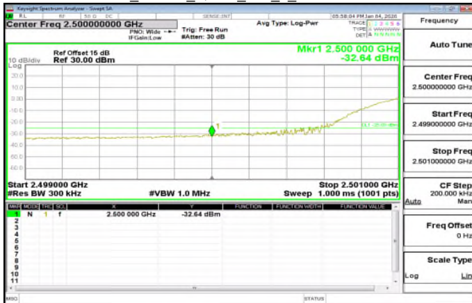
LTE/Band7_20MHz_QPSK_100_0_LowCH20850-2510
