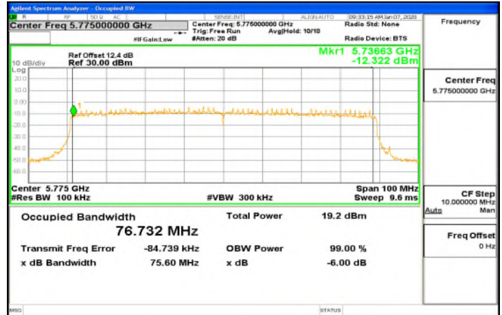
FCC_802.11ax_80MHz_Chain1_5775MHz
