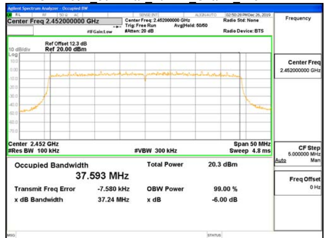
OBW 6dB 802.11ax 40MHz Chain1 2452MHz
