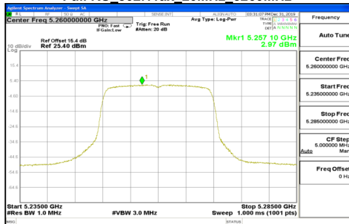
Full RU 802.11ax 20MHz 5260MHz
