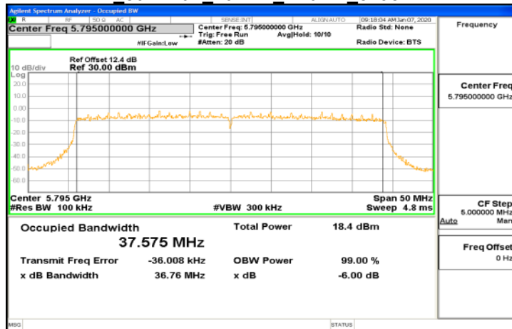
FCC 802.11ax 40MHz Chain1 5795MHz
