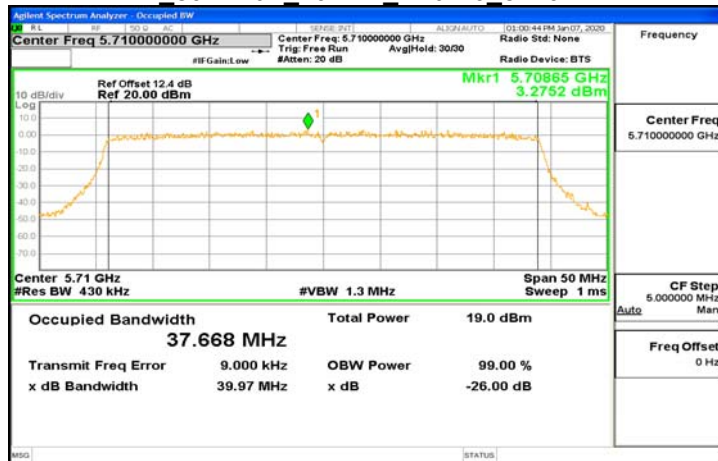
FCC 802.11ax 40MHz Chain0 5710MHz
